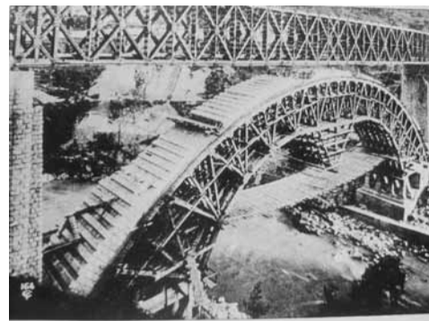
Oder in jeklena konstrukcija
